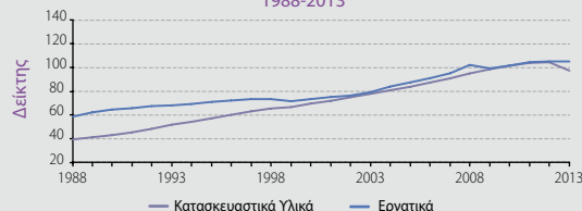
Δείκτες Κόστους στον Τομέα των Κατασκευών (2010=100) 1988-2013
