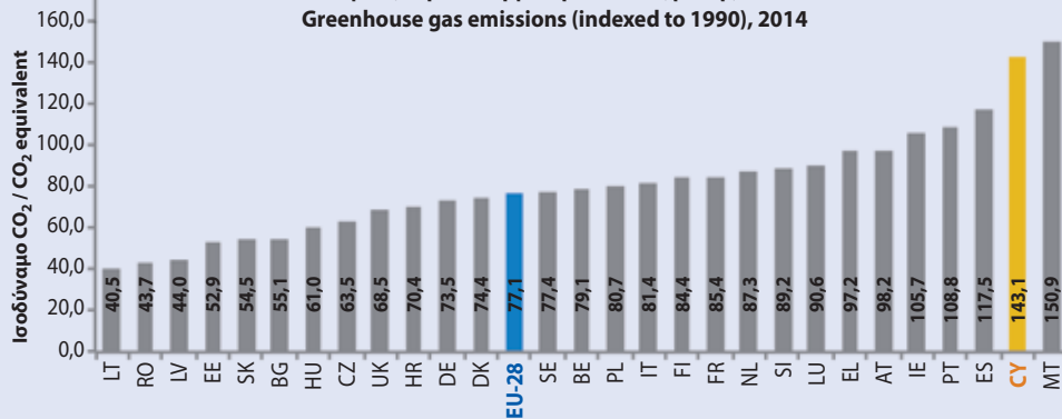
Εκπομπές αερίων θερμοκηπίου (έτος βάσης 1990) / Greenhouse gas emissions (indexed to 1990), 2014
