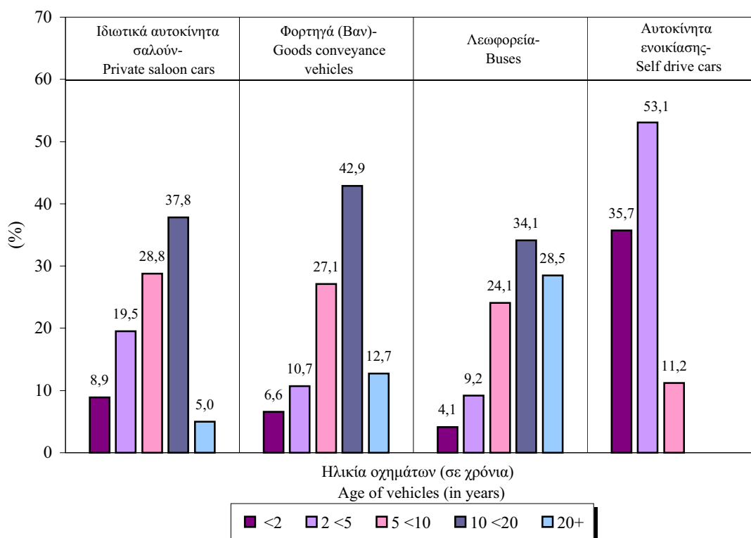
ΔΙΑΓΡΑΜΜΑ 3. ΚΑΤΑΝΟΜΗ ΑΔΕΙΟΥΧΩΝ ΑΥΤΟΚΙΝΗΤΩΝ ΣΤΗΝ ΚΥΠΡΟ ΚΑΤΑ ΗΛΙΚΙΑ, 2009 FIGURE 3. AGE DISTRIBUTION OF LICENSED VEHICLES IN CYPRUS, 2009
