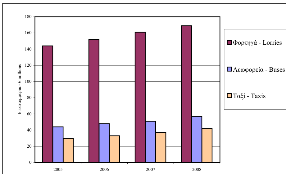
ΔΙΑΓΡΑΜΜΑ 2. ΑΞΙΑ ΠΑΡΑΓΩΓΗΣ ΤΩΝ ΧΕΡΣΑΙΩΝ ΜΕΤΑΦΟΡΩΝ ΚΑΤΑ ΔΡΑΣΤΗΡΙΟΤΗΤΑ, 2005-2008 FIGURE 2. GROSS OUTPUT OF LAND TRANSPORT BY ACTIVITY, 2005-2008
